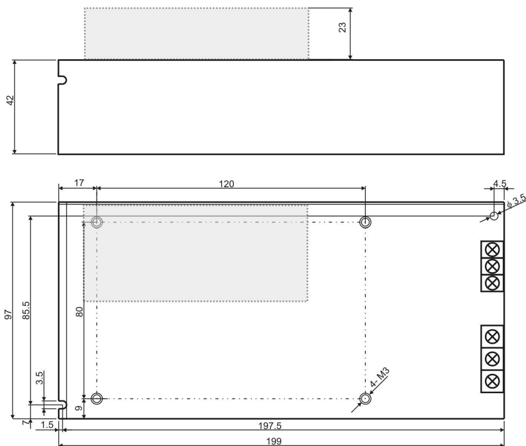
Rysunek 3. Widok mechaniczny zasilacza.
