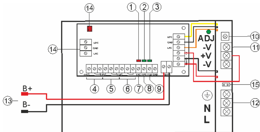
Rys. 2. Widok zasilacza.
