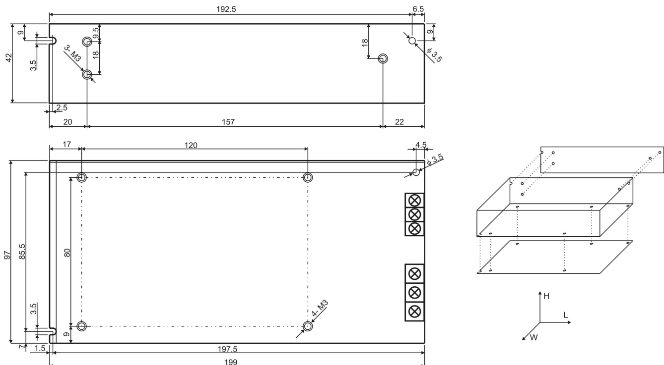
Rysunek 2. Widok mechaniczny zasilacza.
