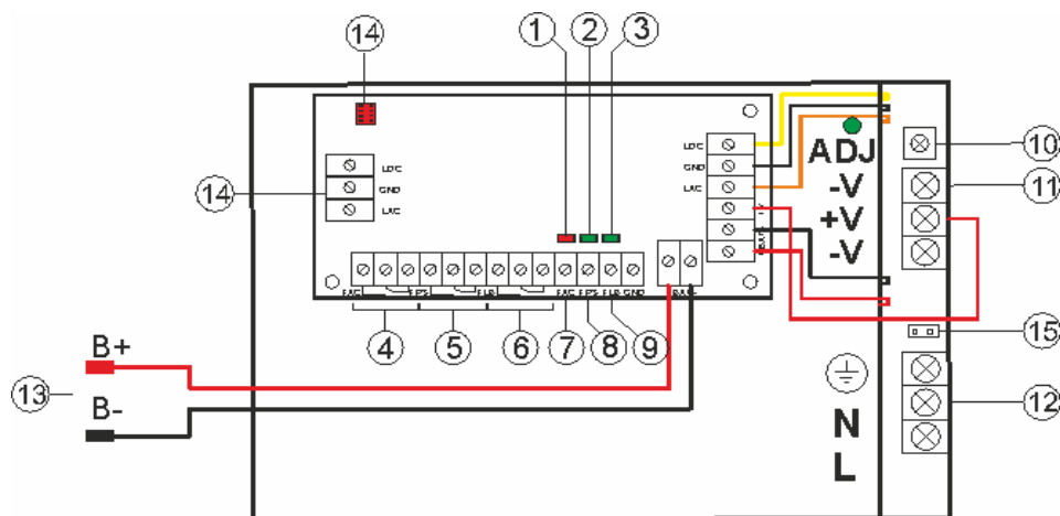
Rysunek. 3. Widok zasilacza z modułem MPSB12.
