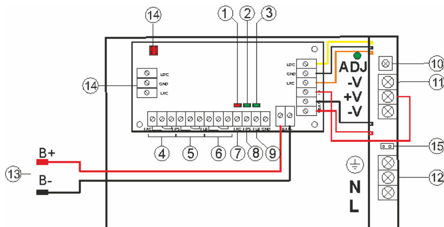
Rysunek. 3. Widok zasilacza z modułem MPSB12.
