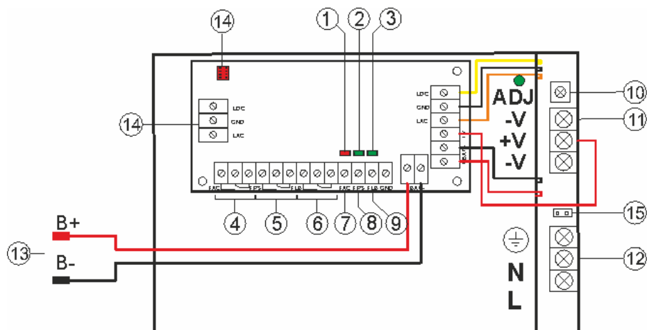
Rysunek. 3. Widok zasilacza z modułem MPSB24.
