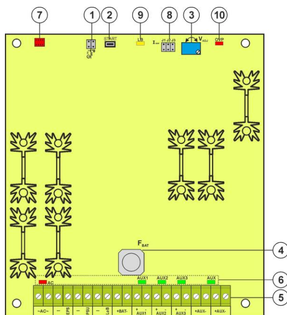
Rys. 2. Widok płyty pcb zasilacza.
