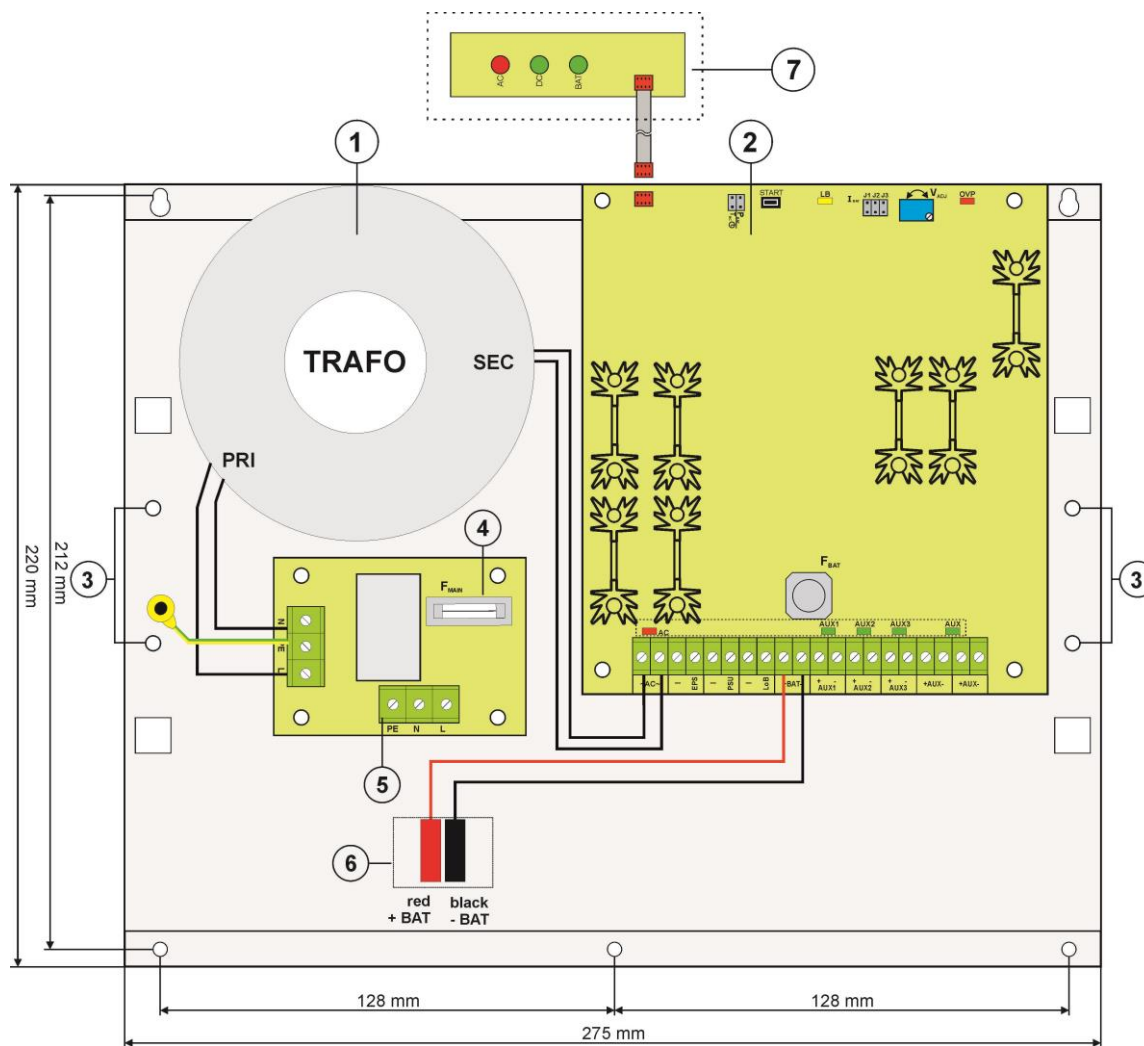
Rys.3. Widok zasilacza.
