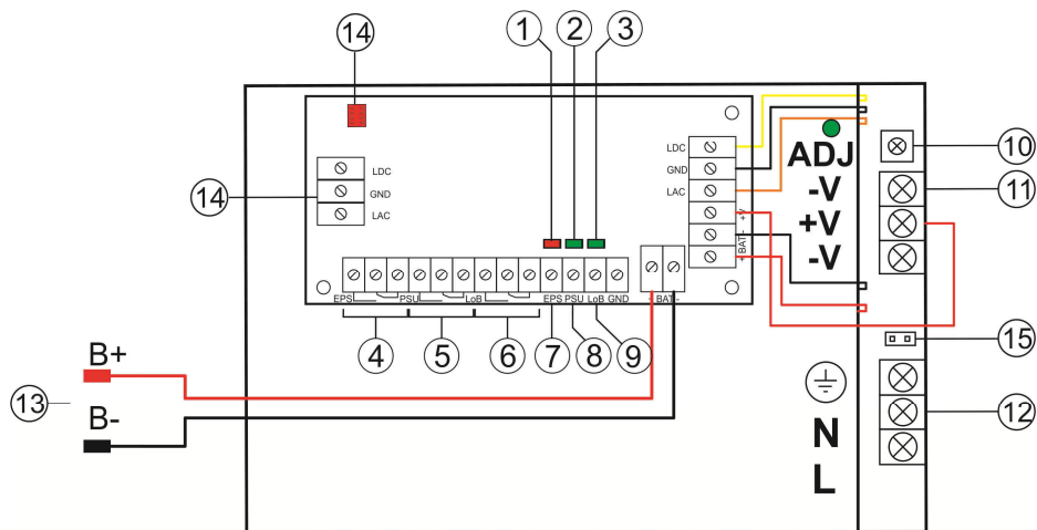
Rys. 2. Widok zasilacza.
