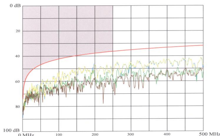
Przykładowy wykres pomiaru PS NEXT kabla U/UTP kategorii 6 produkcji FK MADEX
