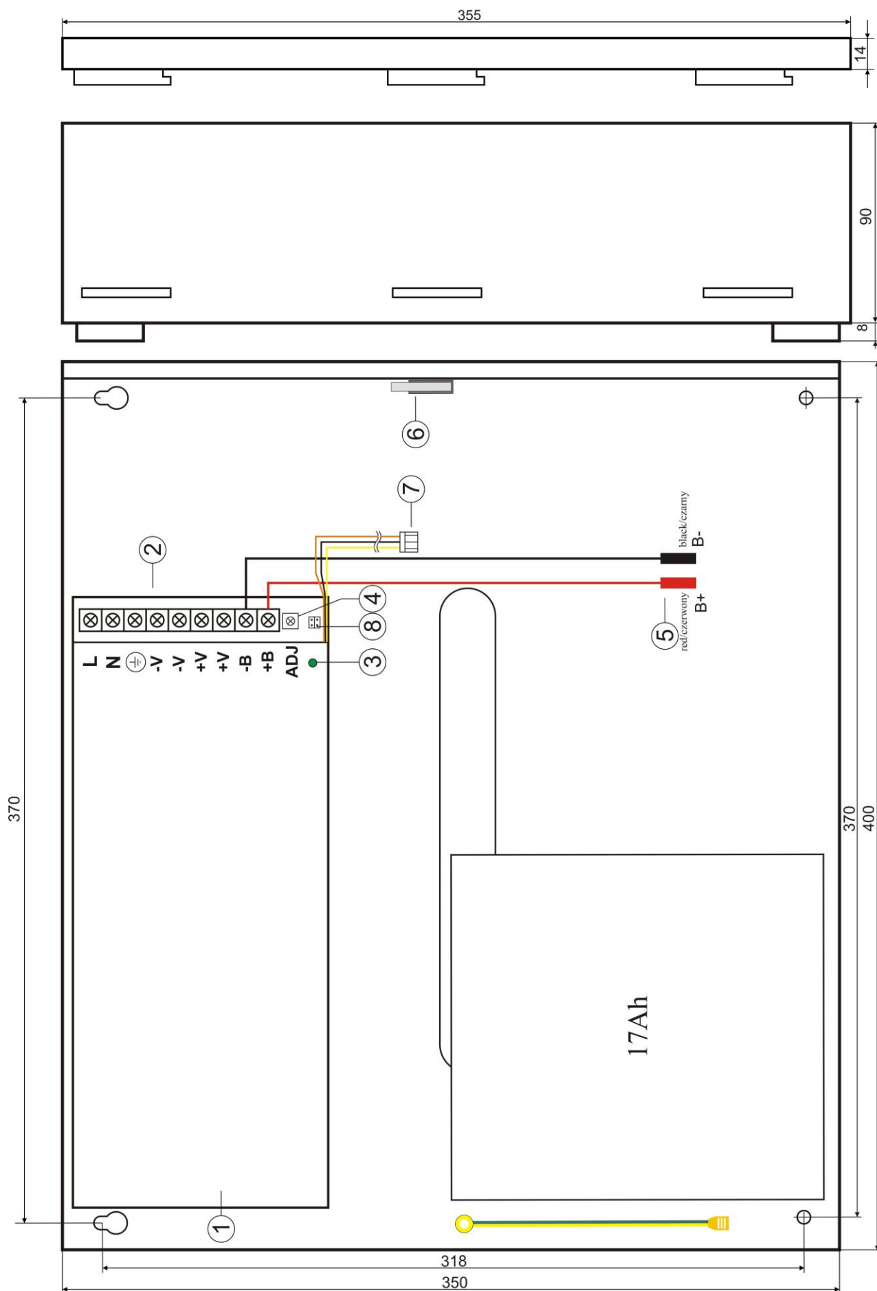
Rys.2. Widok zasilacza.
