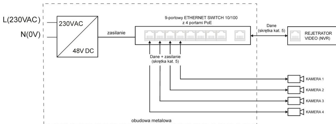
Rys.1. Schemat blokowy.
