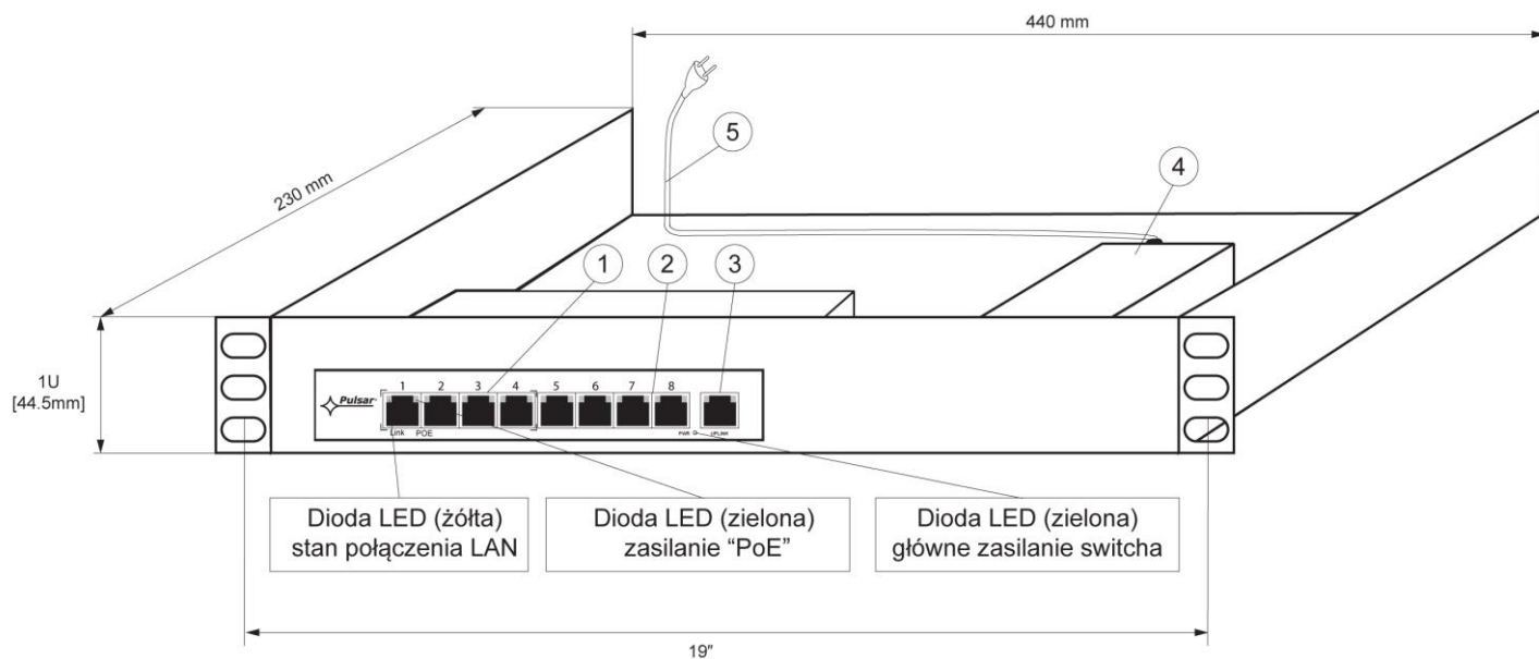
Rys.2. Widok obudowy.
