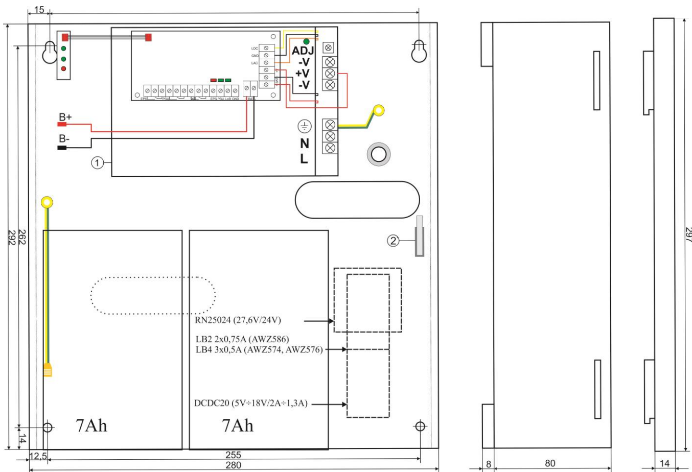
Rys.3. Widok zasilacza.
