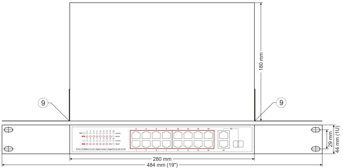
Rys. 4. Widok switch'a.
