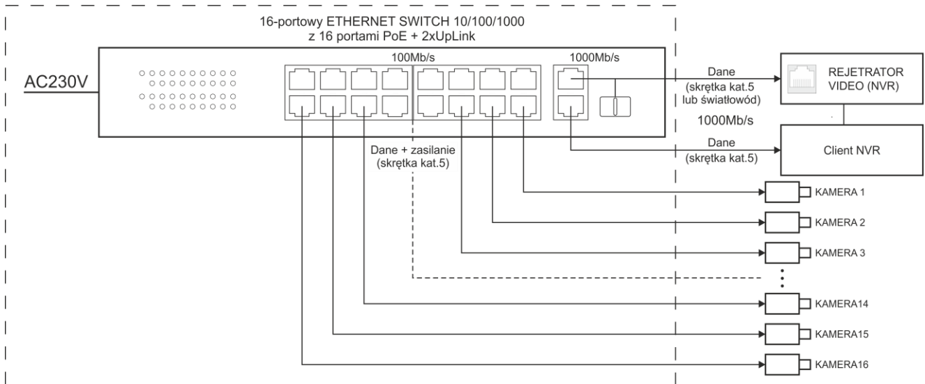
Rys. 1. Schemat blokowy.
