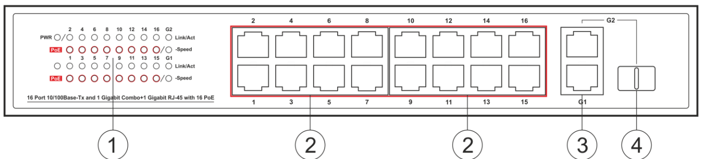
Rys. 2. Panel czołowy switcha.
