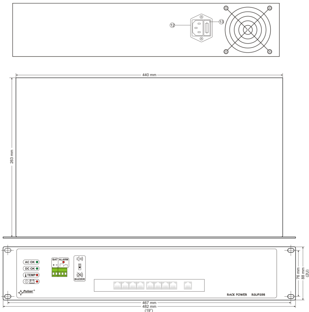
Rys.3. Widok zasilacza.
