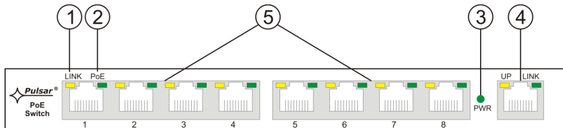
Rys. 4. Widok Switch'a.
