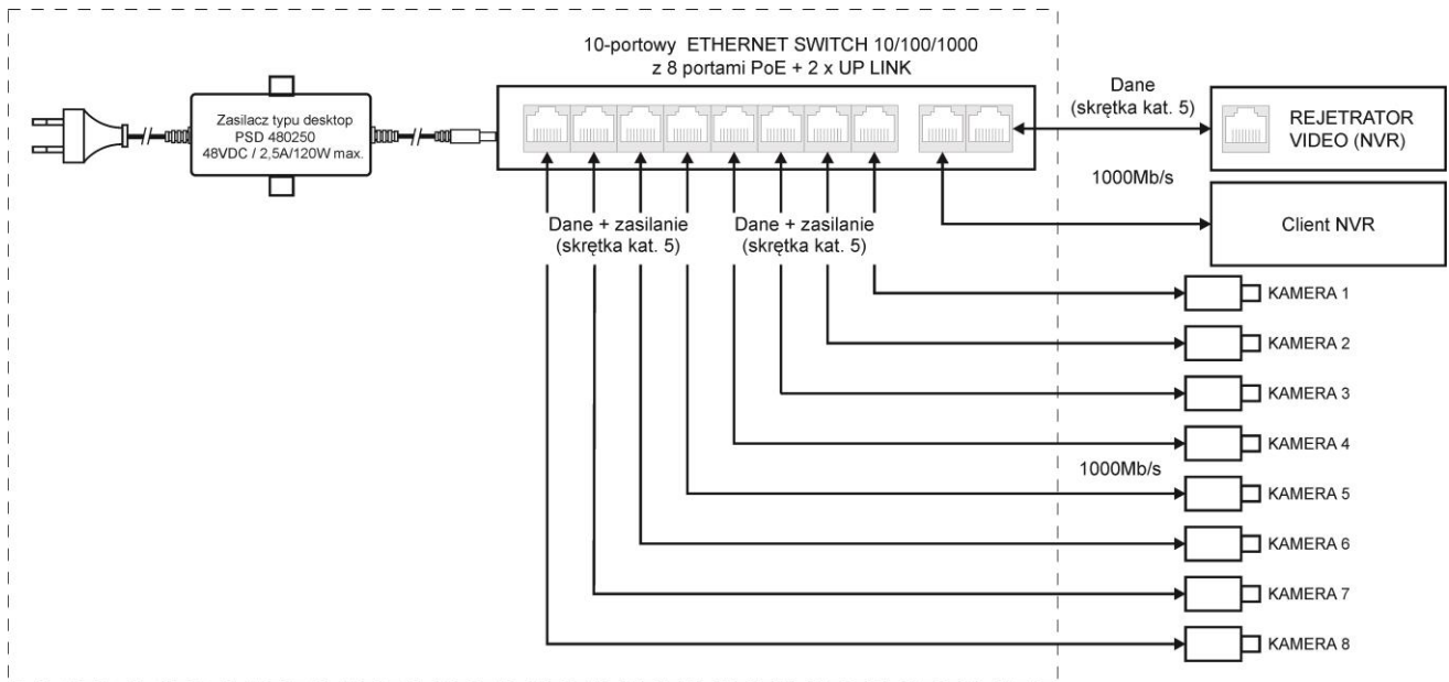
Rys. 1. Schemat blokowy.
