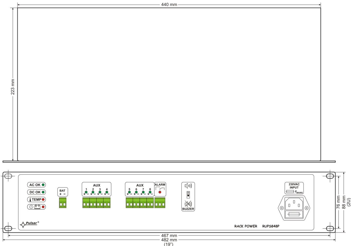
Rys.3. Widok zasilacza.
