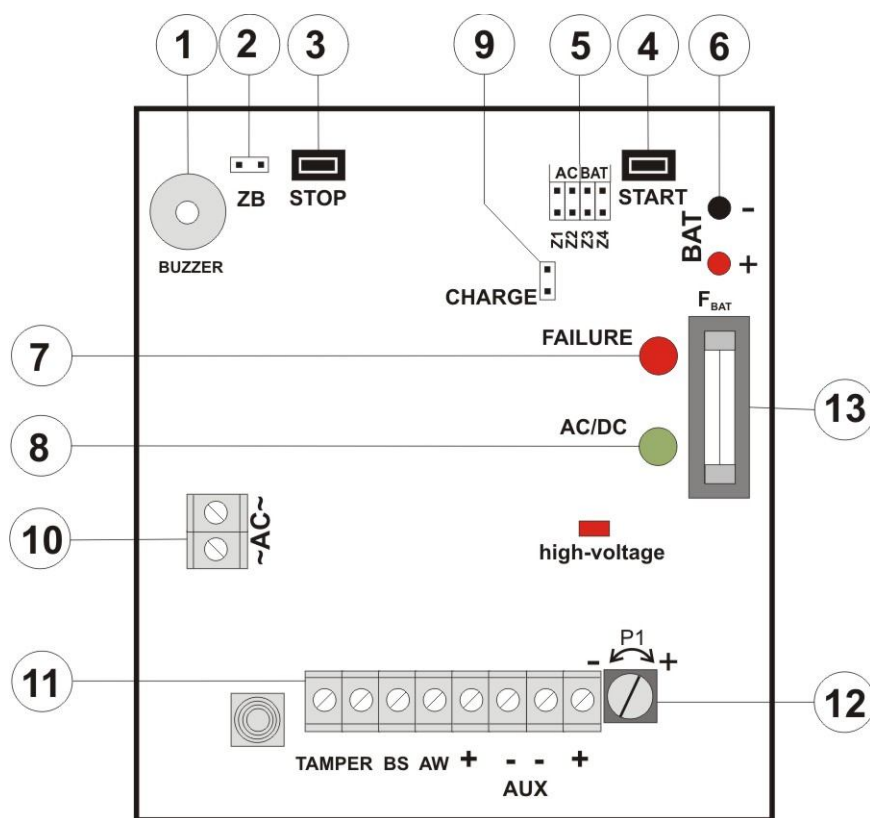
Rys. 2. Widok płyty pcb zasilacza.
