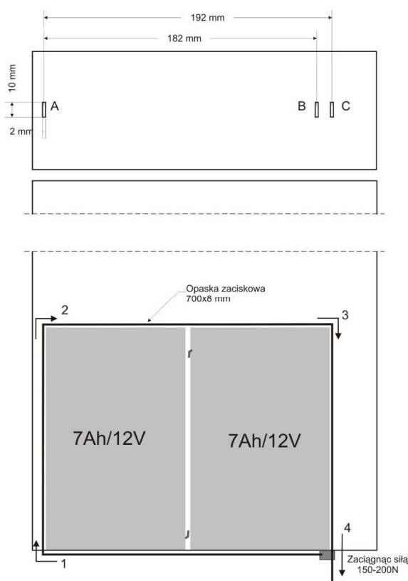
Rys.5. Procedura mocowania akumulatorów.
