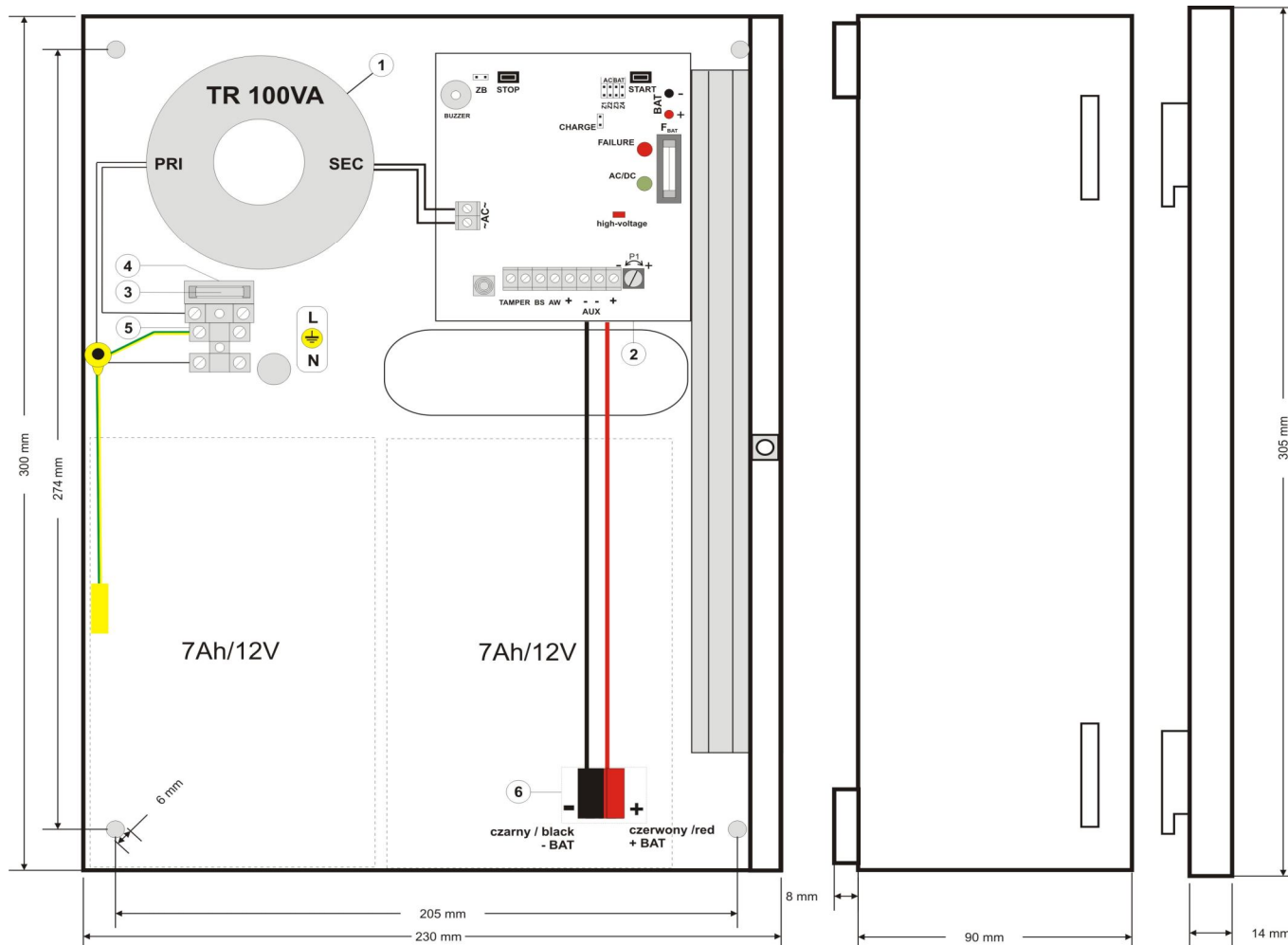
Rys.3. Widok zasilacza.
