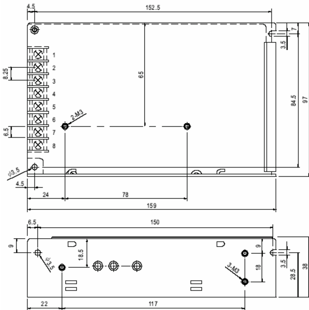
Rys 1. Gabaryty oraz sposób mocowania zasilacza AD55
