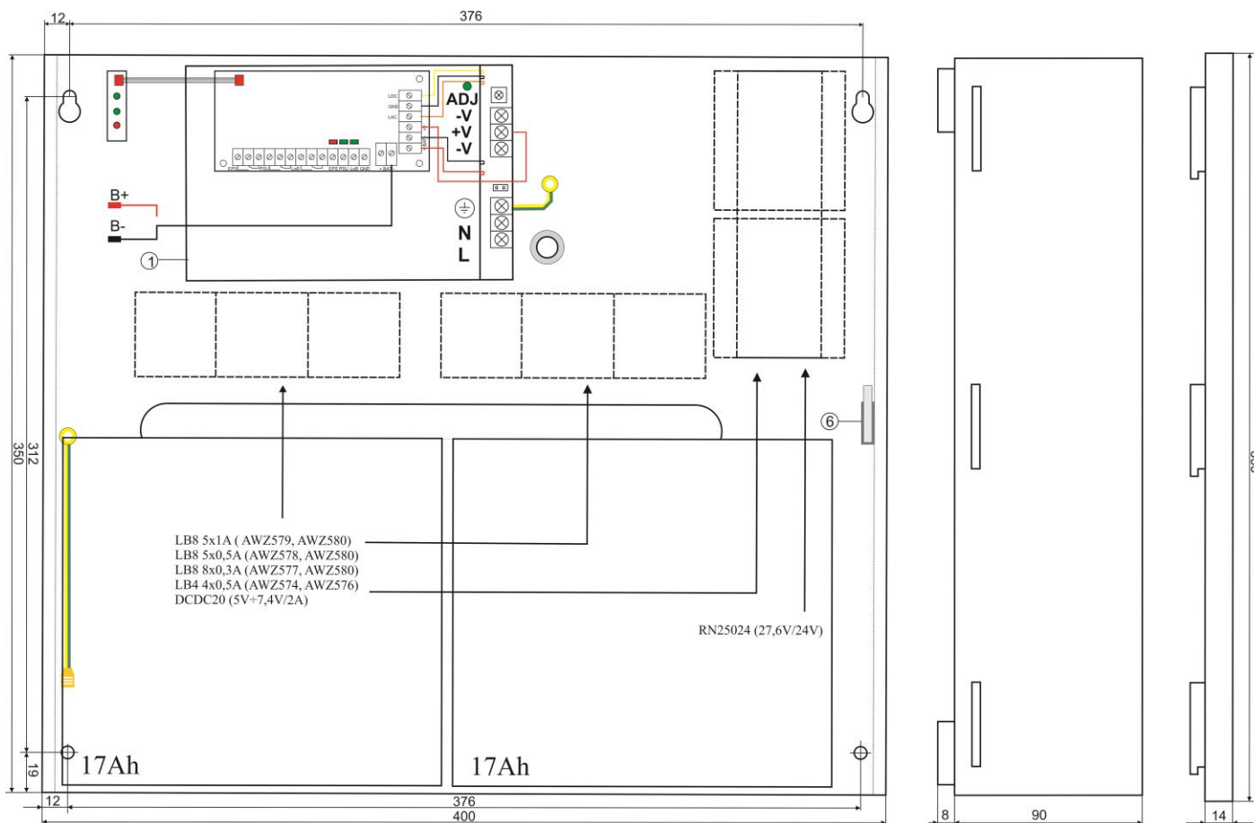
Rys.3. Widok zasilacza.
