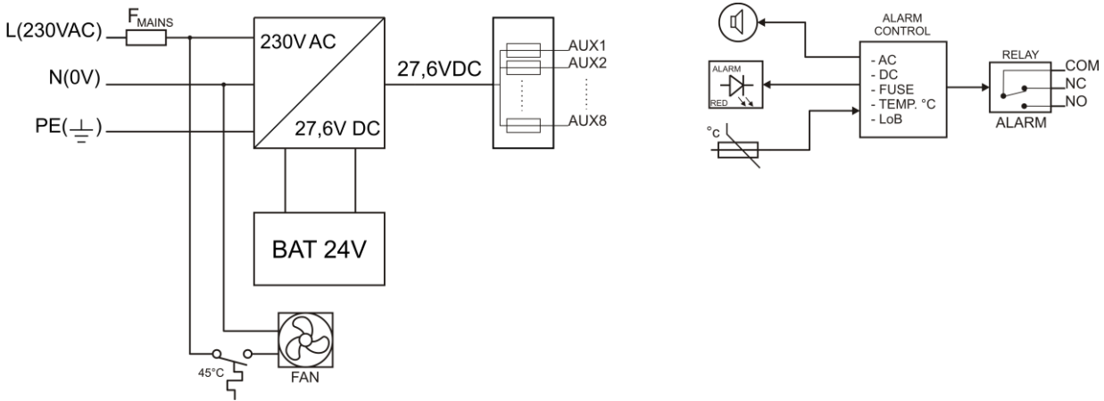
Rys.1. Schemat blokowy zasilacza.
