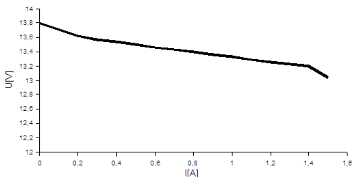
Rys. 4. Charakterystyka prądowo-napięciowa zasilacza.
