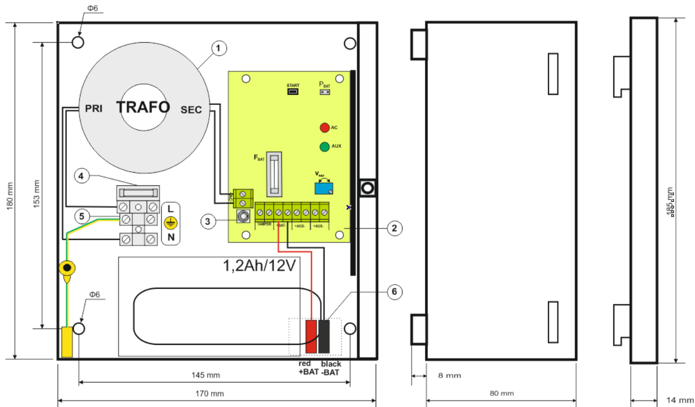
Rys.3. Widok zasilacza.
