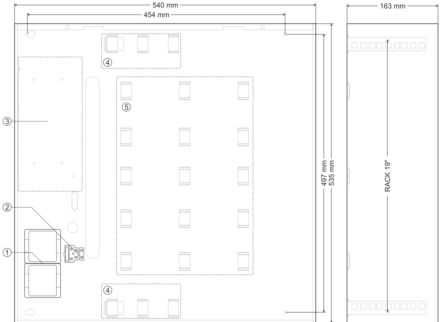
Rys.1 Widok obudowy
