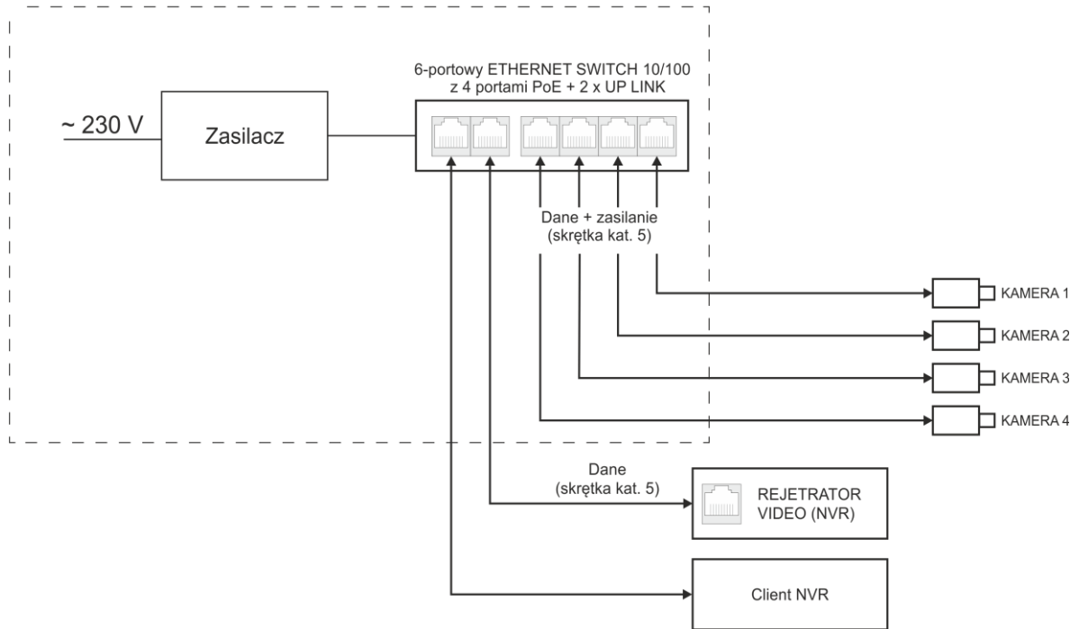
Rys. 1. Schemat blokowy.
