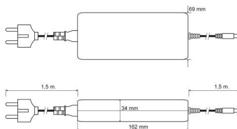
Rys.1. Widok mechaniczny zasilacza.
